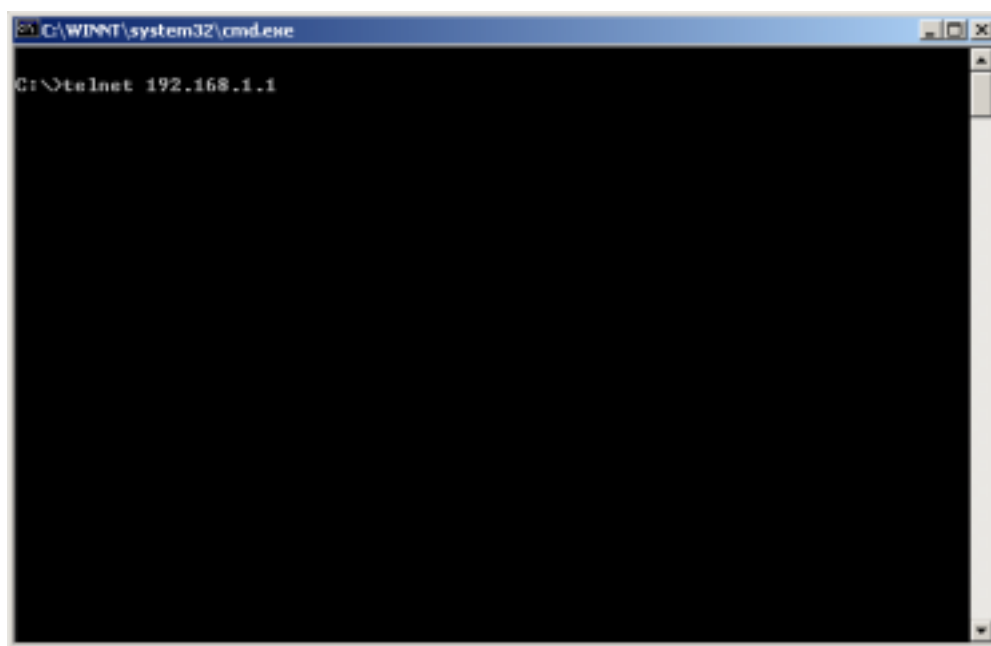
图 4-13 启动Telnet
